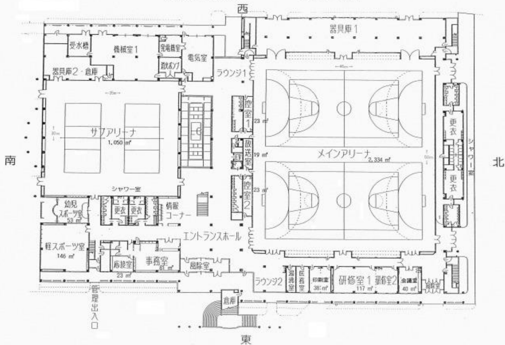
1 階平面図
