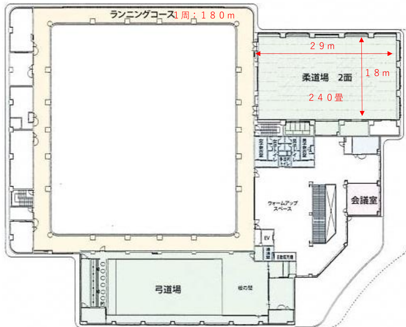
N C V ふくしまアリーナ 2 階平面図
